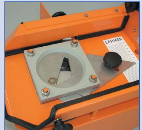
Die Durchflussmenge kann am Dosierschieber stufenlos eingestellt werden.
