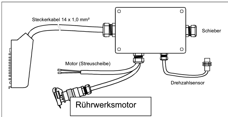
Schaltplan Verteilerkasten
